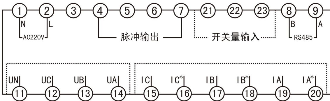
96*96 尺寸后面端子示意图
