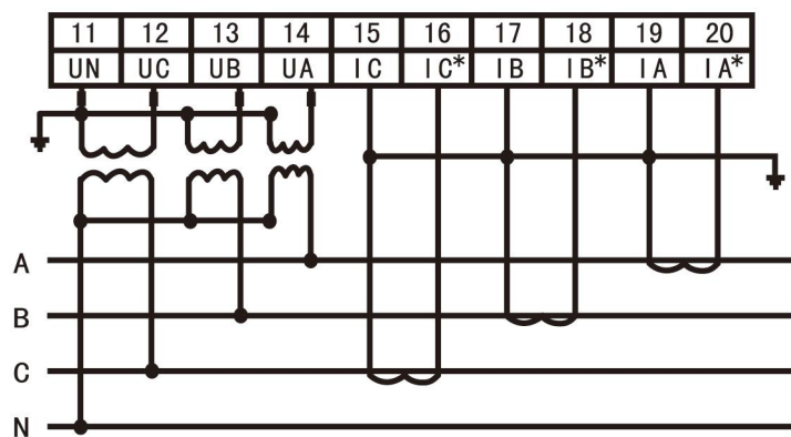
电压经互感器接入、电流经互感器接入
