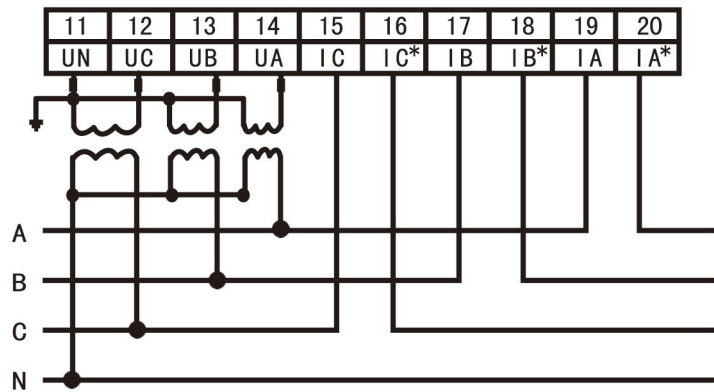
电压经互感器接入、电流直接接入
