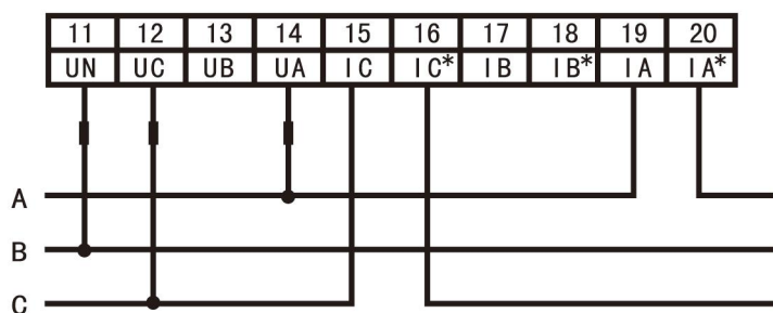
电压直接接入、电流直接接入
