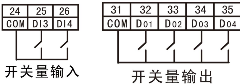
96*96 尺寸后面端子示意图
